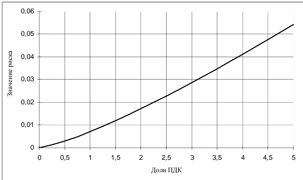
Рис. 4. Потенциальный риск развития хронических эффектов при воздействии фенола
