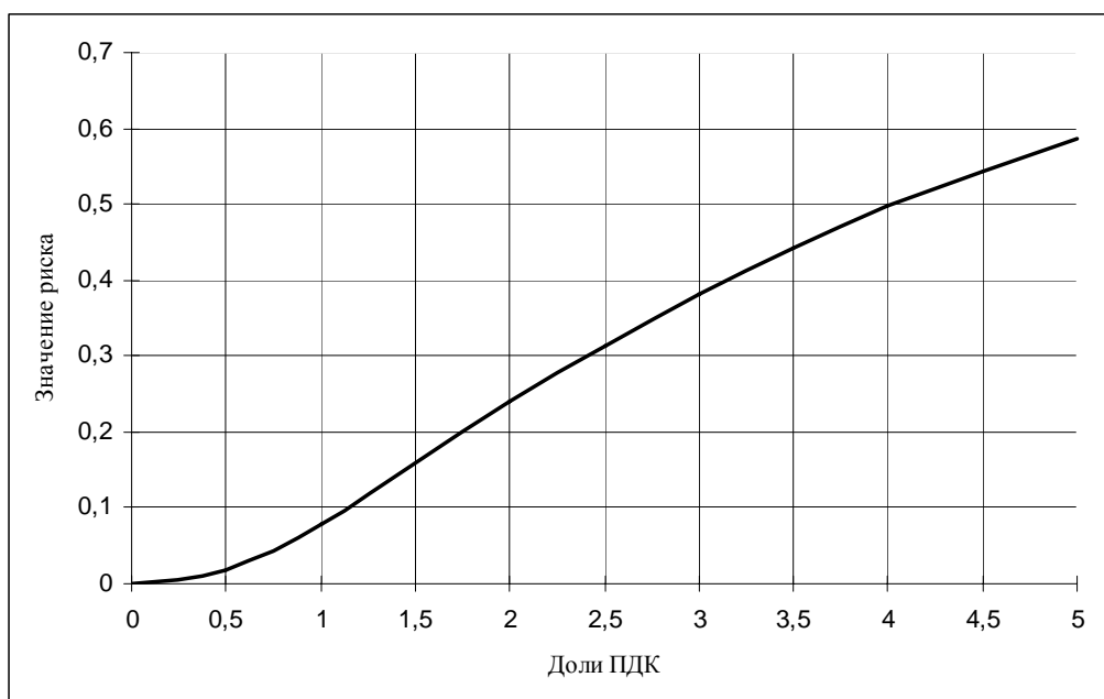
Рис. 17. Потенциальный риск развития рефлекторных эффектов при воздействии углерода оксида
