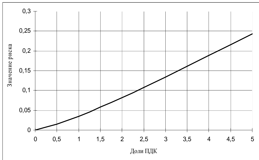
Рис. 8. Потенциальный риск развития хронических эффектов при воздействии формальдегида
