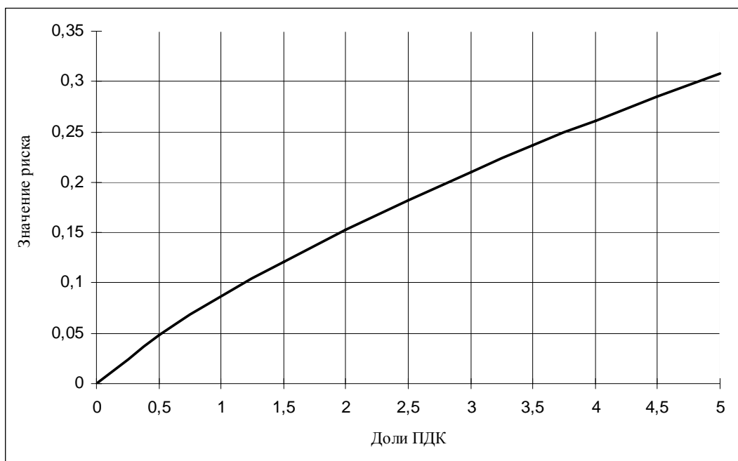
Рис. 18. Потенциальный риск развития хронических эффектов при воздействии углерода оксида
