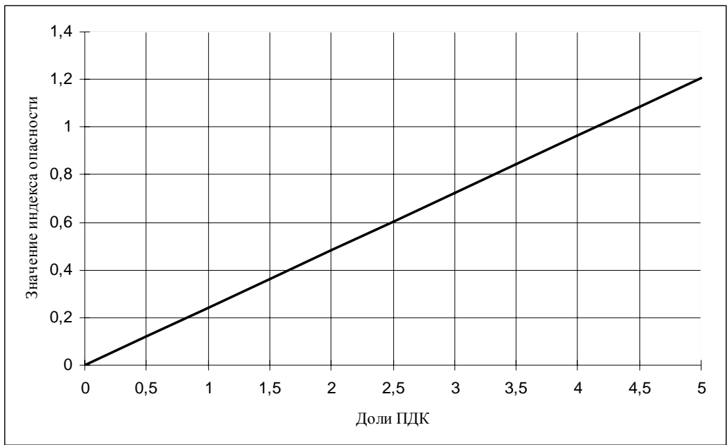
Рис. 9 — Коэффициент опасности при кратковременном воздействии формальдегида
