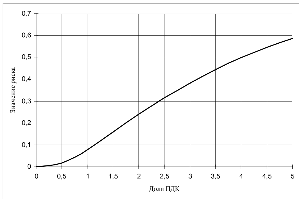
Рис. 1. Потенциальный риск развития рефлекторных эффектов при воздействии аммиака
