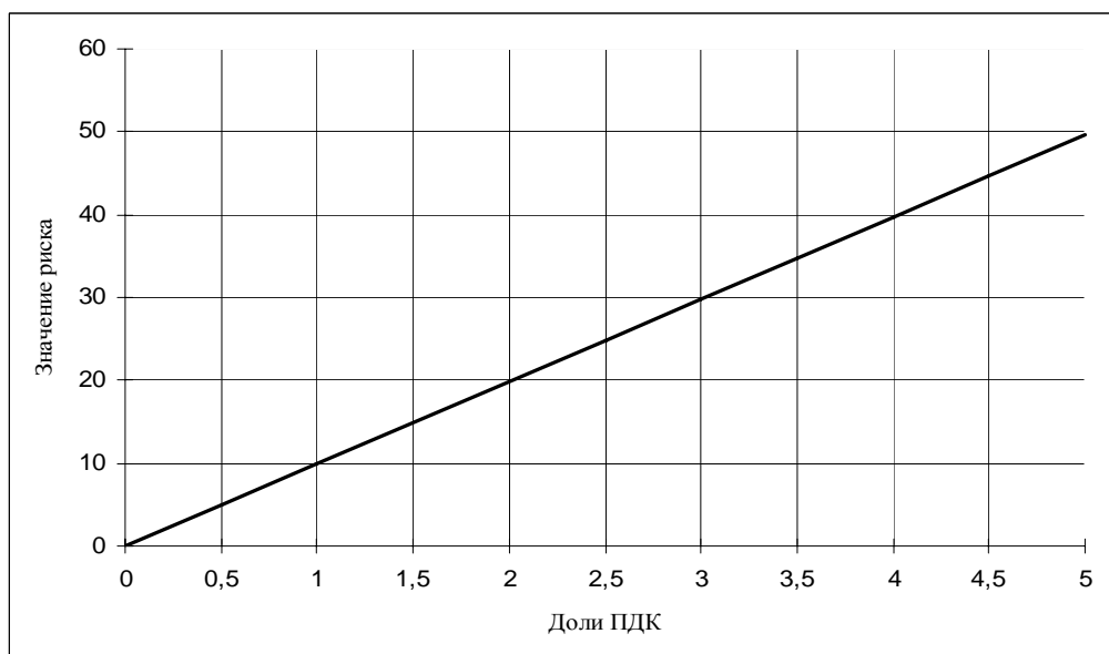
Рис. 12. Популяционный канцерогенный риск при воздействии формальдегида (дополнительных случаев в течение жизни на 1 000 000 человек)
