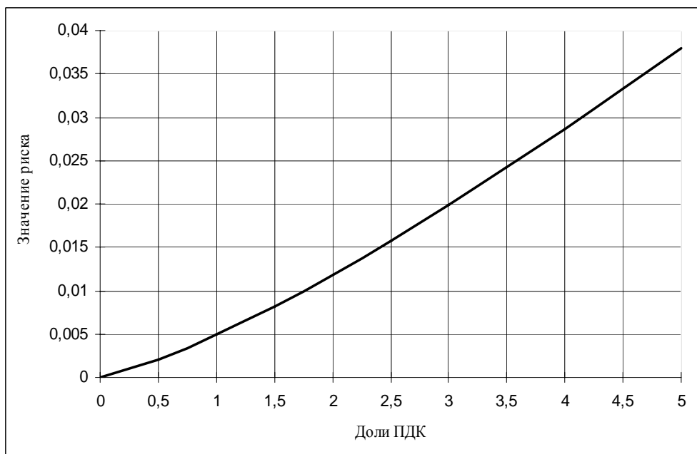
Рис. 14. Потенциальный риск развития хронических эффектов при воздействии азота диоксида
