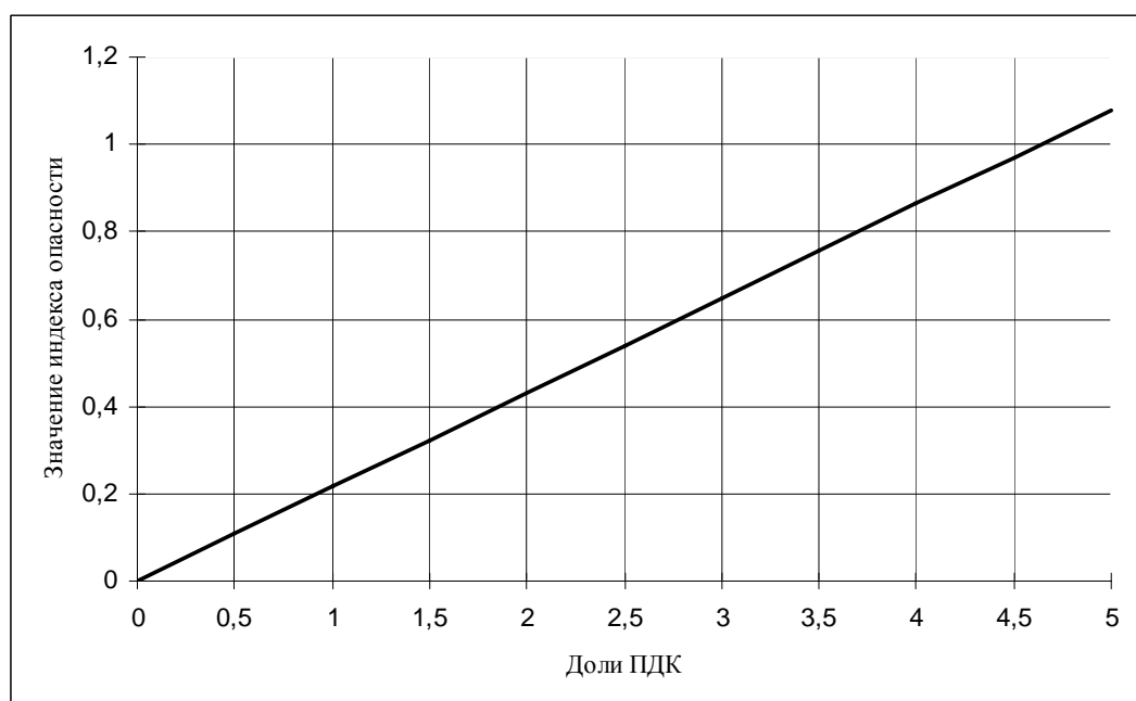
Рис. 2. Коэффициент опасности при кратковременном воздействии аммиака
