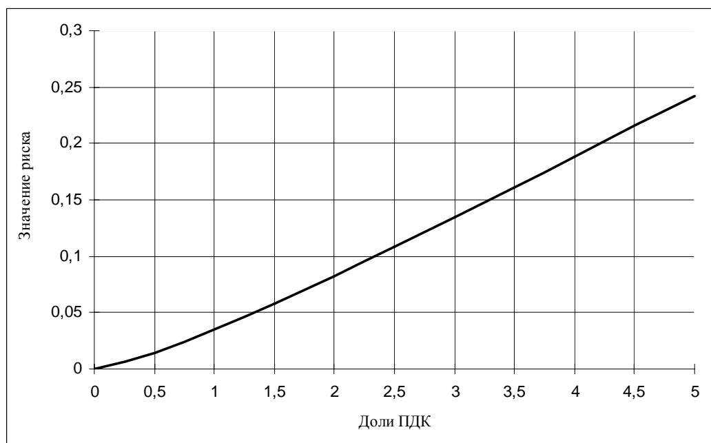
Рис. 8. Потенциальный риск развития хронических эффектов при воздействии формальдегида
