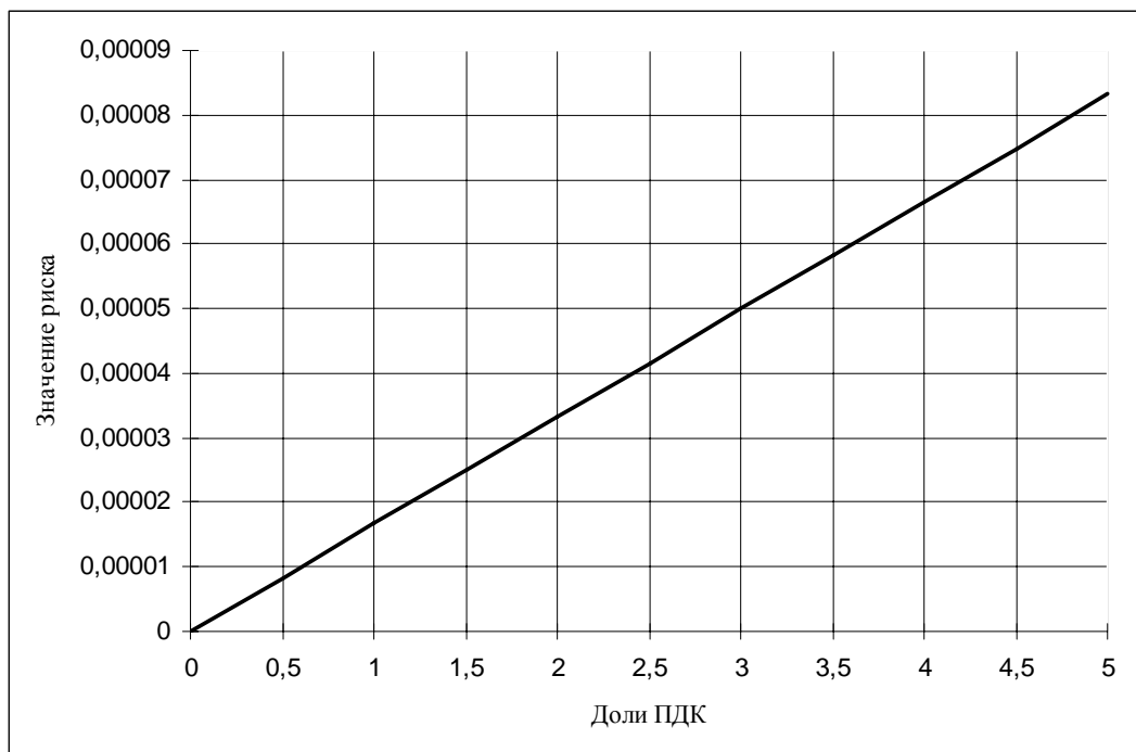
Рис. 25. Индивидуальный канцерогенный риск при воздействии бензола
