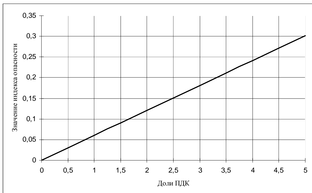
Рис. 16. Коэффициент опасности при хроническом воздействии азота диоксида
