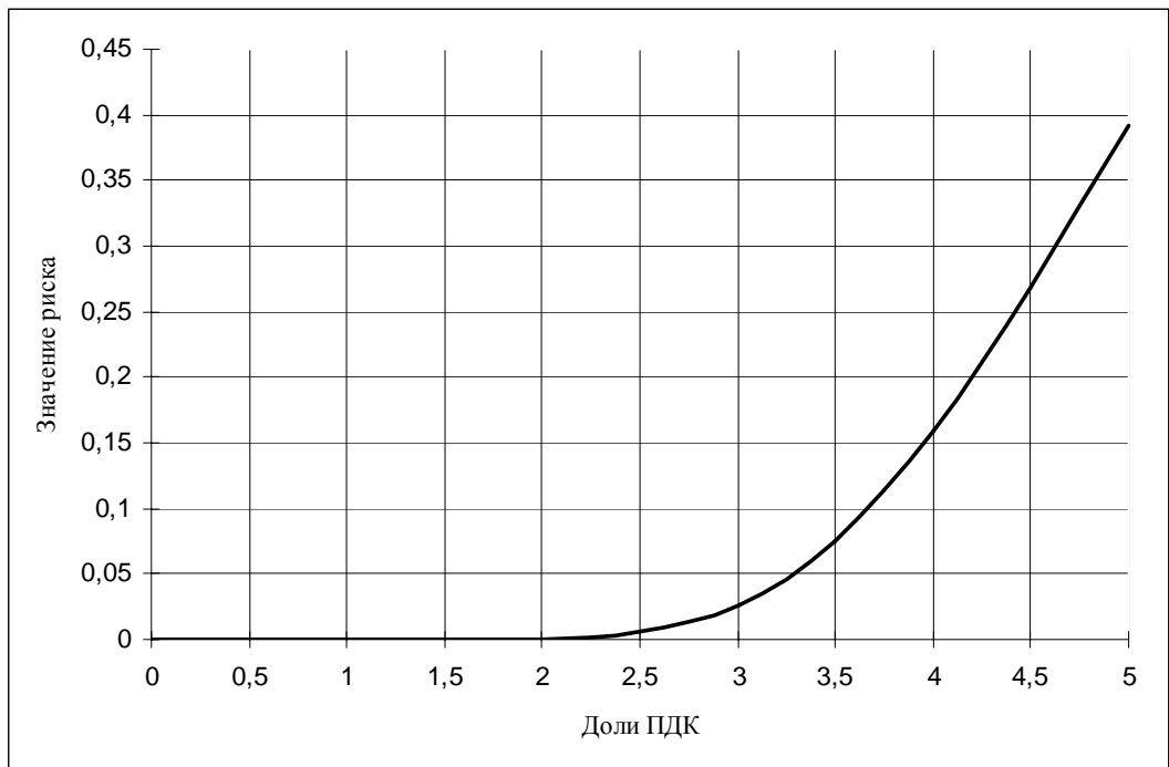
Рис. 3. Потенциальный риск развития рефлекторных эффектов при воздействии фенола
