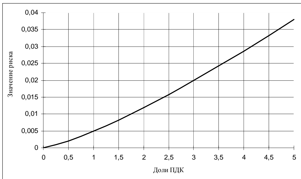
Рис. 14. Потенциальный риск развития хронических эффектов при воздействии азота диоксида
