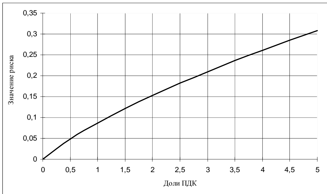
Рис. 18. Потенциальный риск развития хронических эффектов при воздействии углерода оксида
