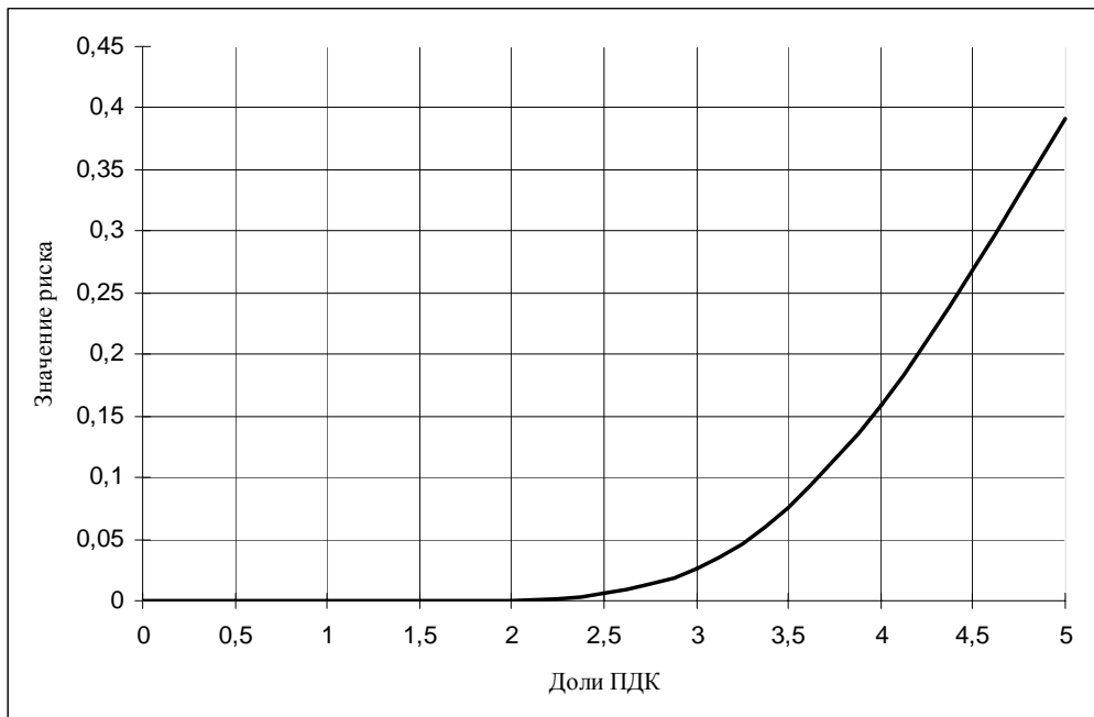
Рис. 13. Потенциальный риск развития рефлекторных эффектов при воздействии азота диоксида
