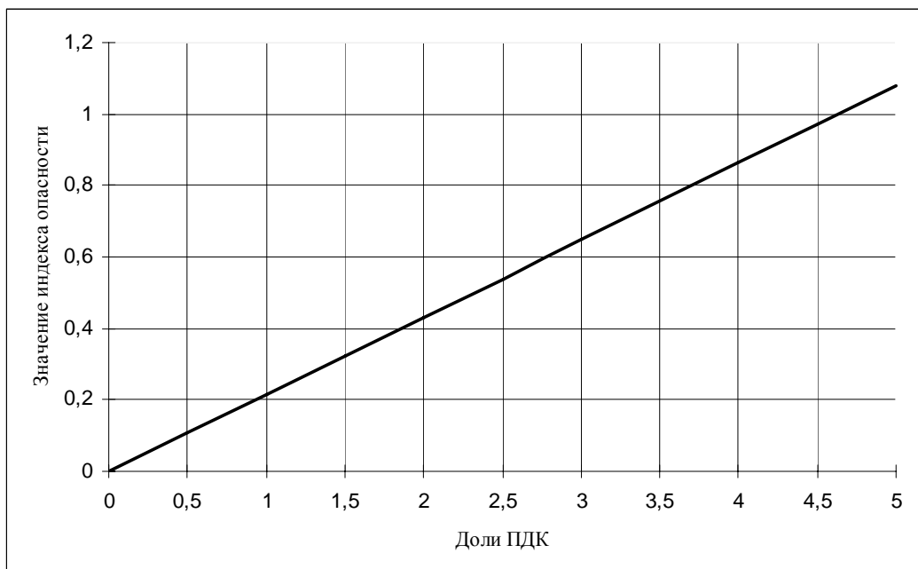
Рис. 23. Коэффициент опасности при кратковременном воздействии бензола
