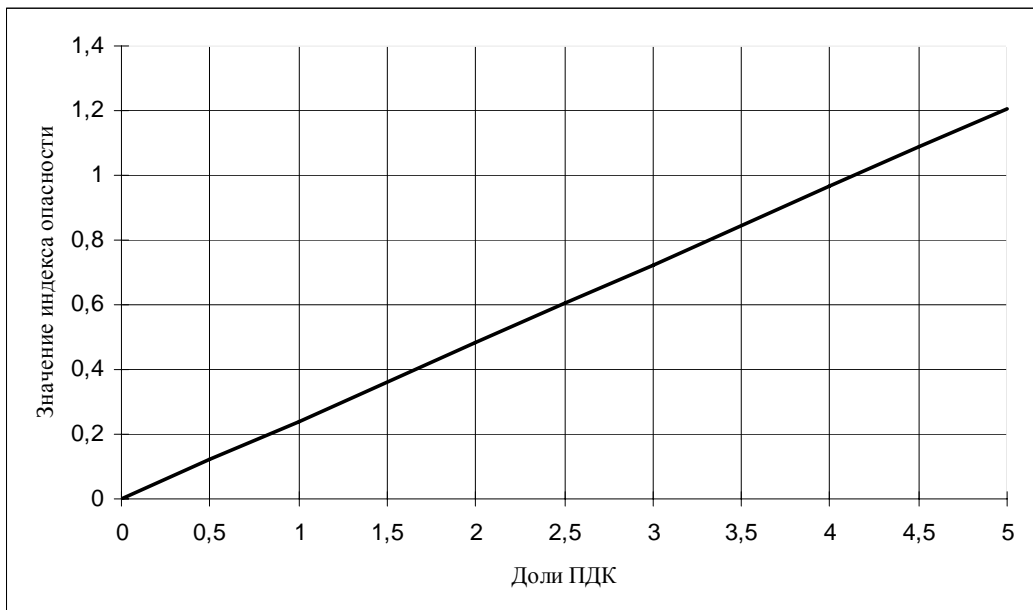
Рис. 5. Коэффициент опасности при кратковременном воздействии фенола
