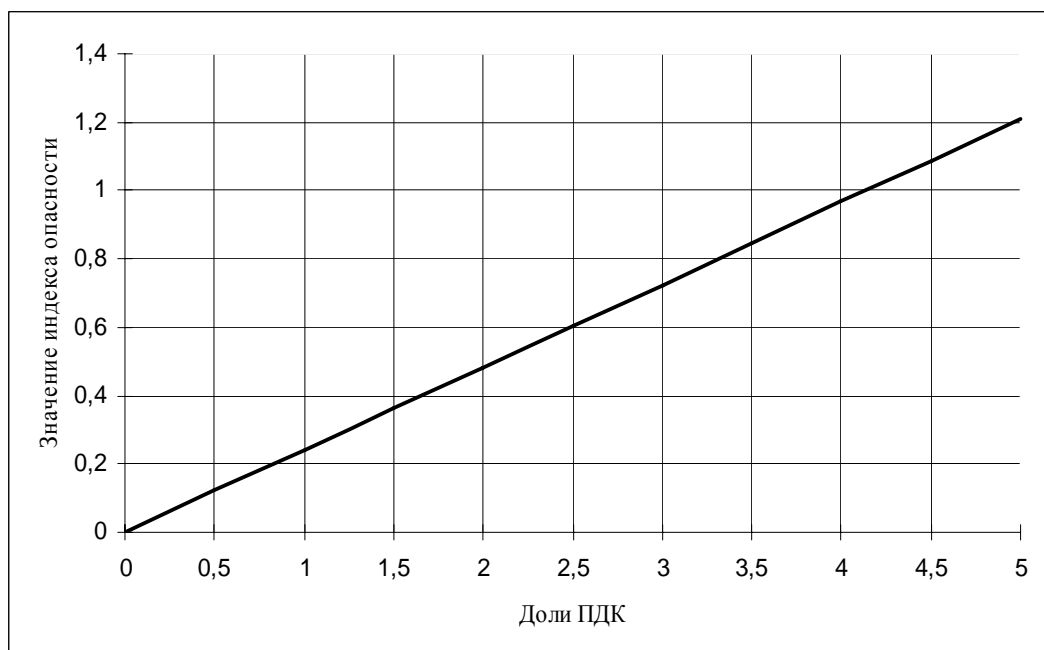
Рис. 24. Коэффициент опасности при хроническом воздействии бензола
