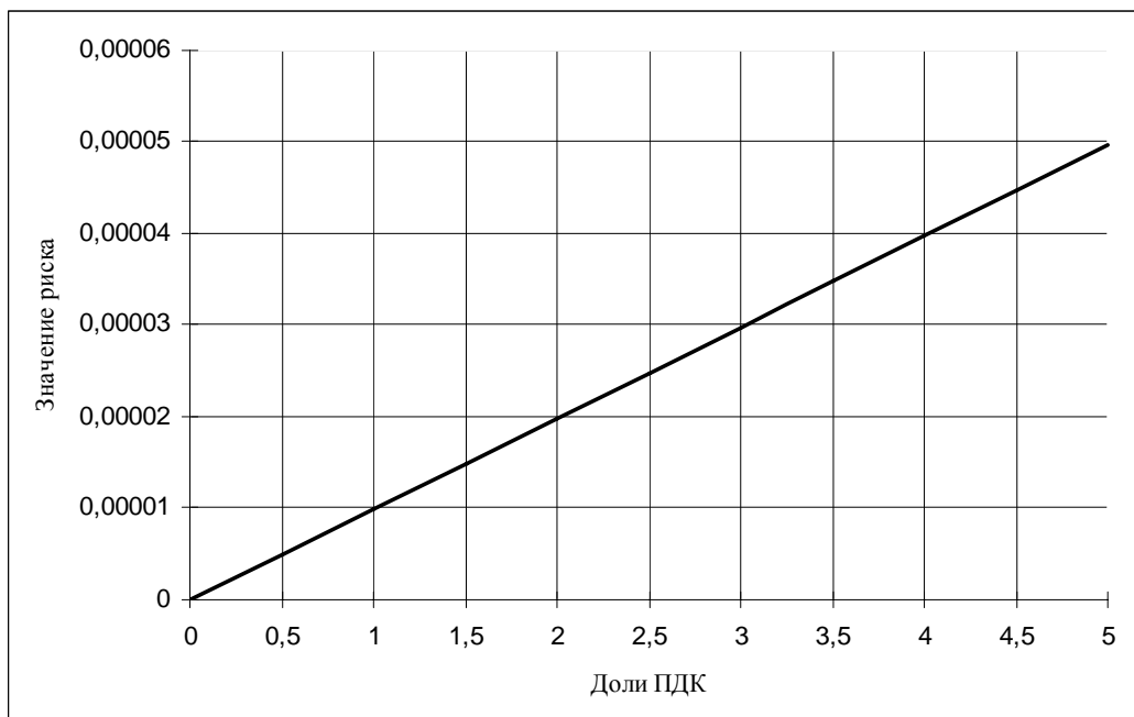
Рис. 11. Индивидуальный канцерогенный риск при воздействии формальдегида
