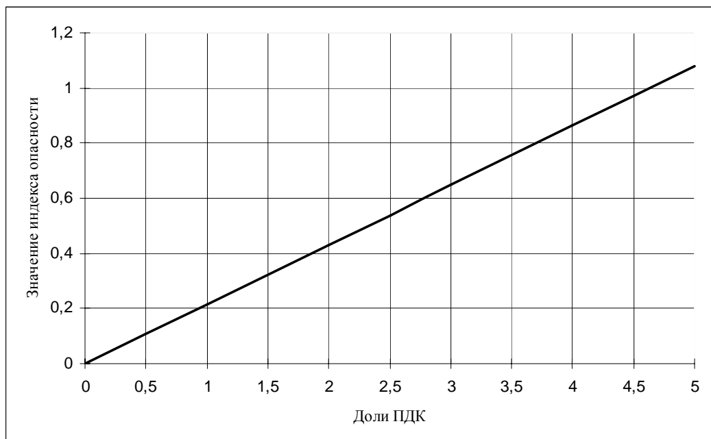
Рис. 15. Коэффициент опасности при кратковременном воздействии азота диоксида
