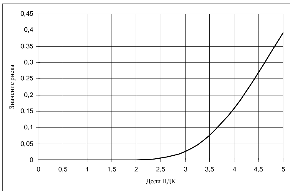
Рис. 7. Потенциальный риск развития рефлекторных эффектов при воздействии формальдегида
