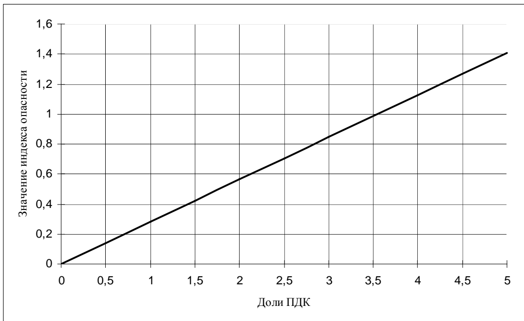
Рис. 10. Коэффициент опасности при хроническом воздействии формальдегида
