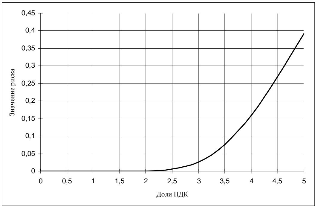
Рис. 21. Потенциальный риск развития рефлекторных эффектов при воздействии бензола
