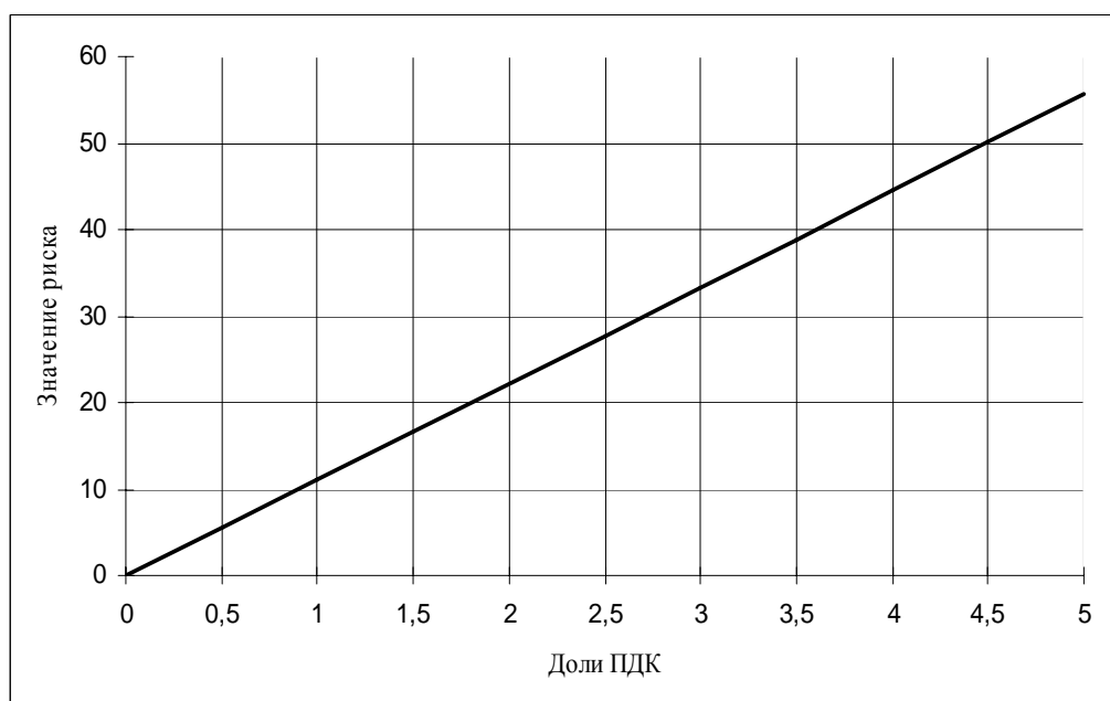
Рис. 12— Популяционный канцерогенный риск при воздействии формальдегида (дополнительных случаев в течение жизни на 1 000 000 человек)
