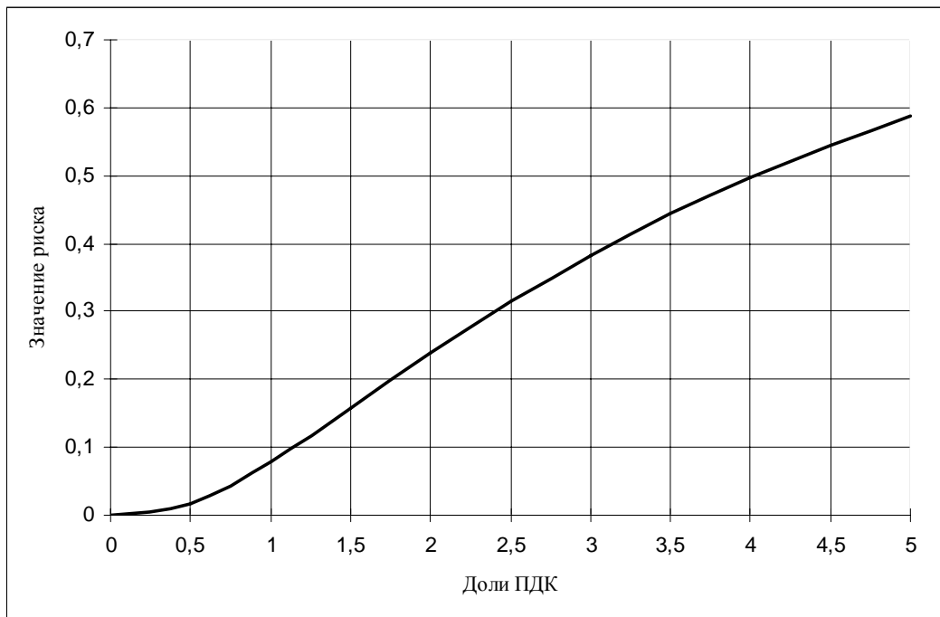
Рис. 17. Потенциальный риск развития рефлекторных эффектов при воздействия углерода оксида
