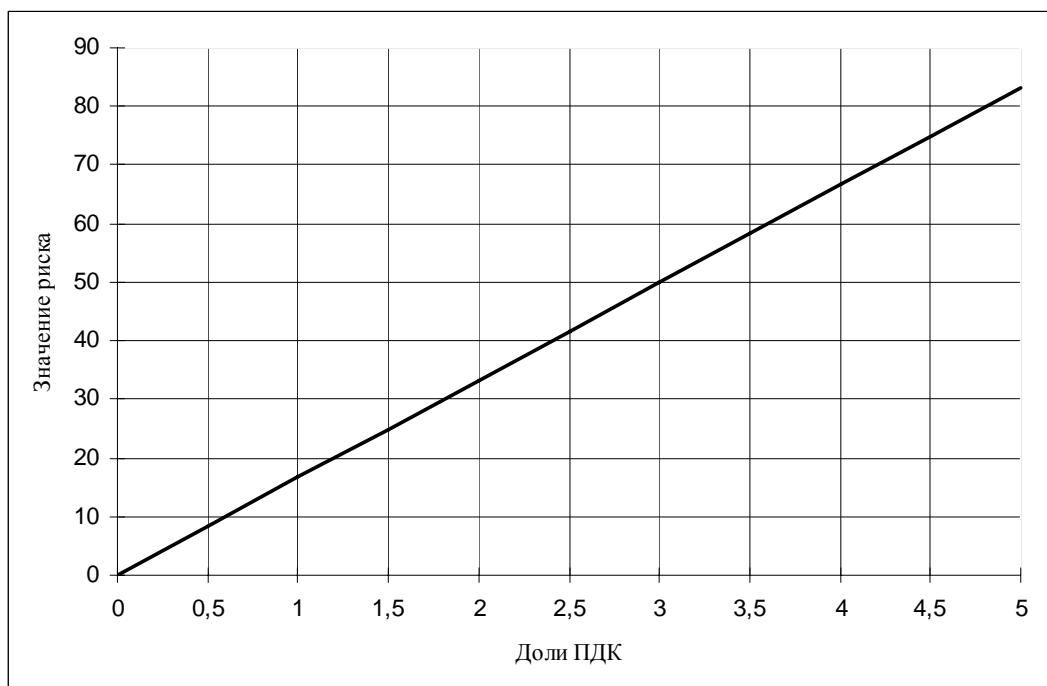
Рис. 26. Популяционный канцерогенный риск при воздействии бензола (дополнительных случаев в течение жизни на 1 000 000 человек)
