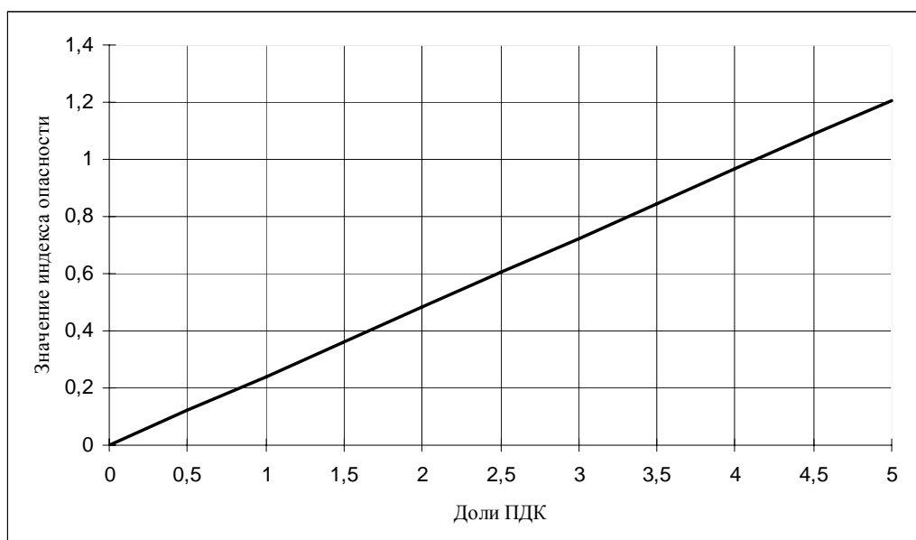
Рис. 15. Коэффициент опасности при кратковременном воздействии азота диоксида
