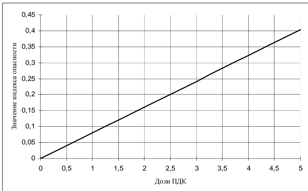
Рис. 6. Коэффициент опасности при хроническом воздействии фенола
