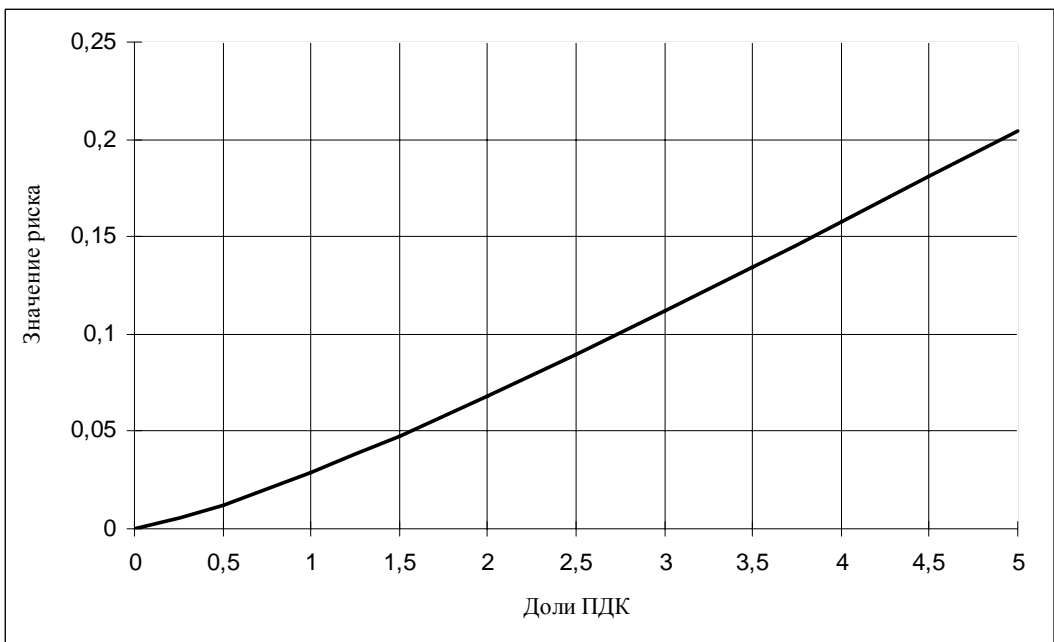
Рис. 22. Потенциальный риск развития хронических эффектов при воздействии бензола
