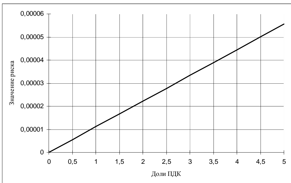
Рис. 11. Индивидуальный канцерогенный риск при воздействии формальдегида
