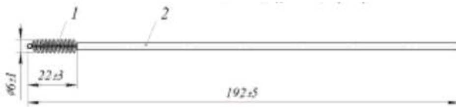
Рисунок 1. – Цитощетка: 1 – рабочая часть, 2 – рукоятка
